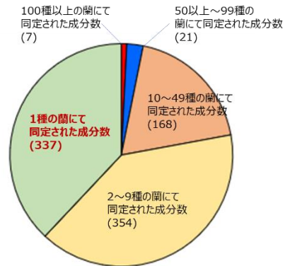
図 2 機器分析により同定された887の香気成分頻出度合
